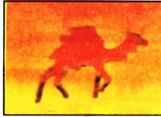
جَمَل
